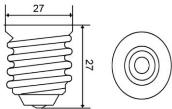
E27 / E26 ES / PAR30 or PAR38
